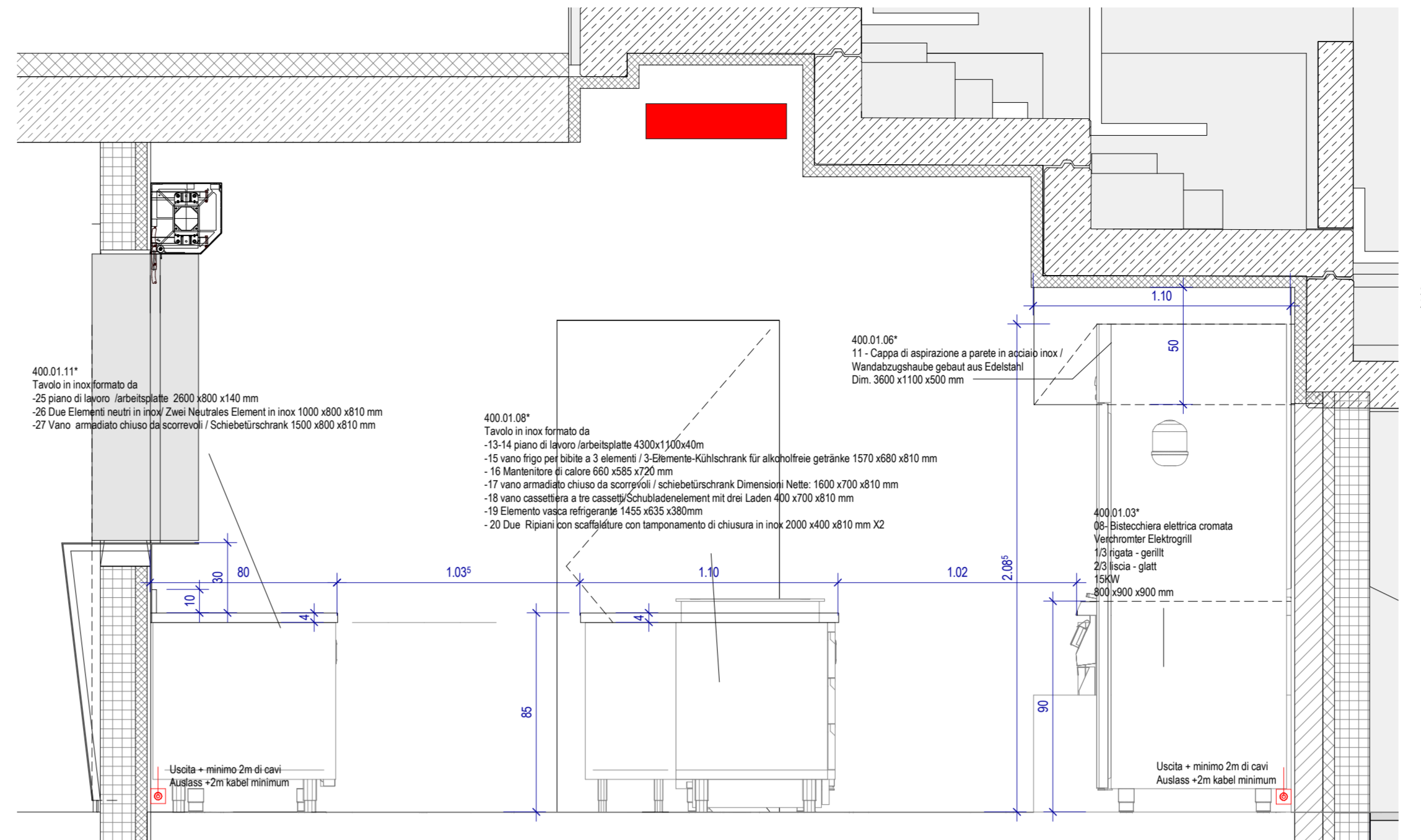
Sezione BB cucina chiosco - Schnitt BB küche kiosk
