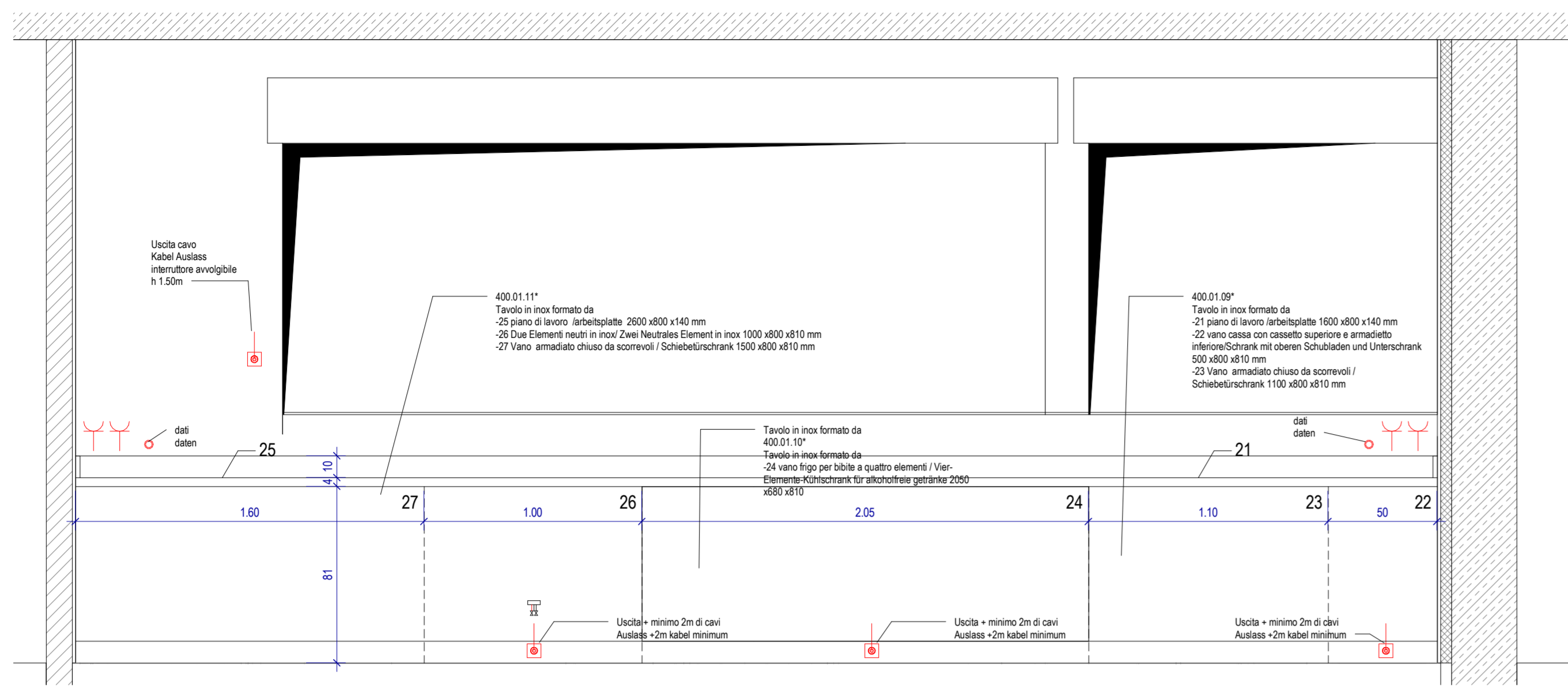
Sezione CC cucina chiosco - Schnitt CC küche kiosk
